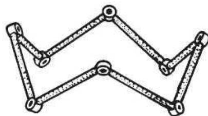
Abbildung 1 Schwefelmolekül
